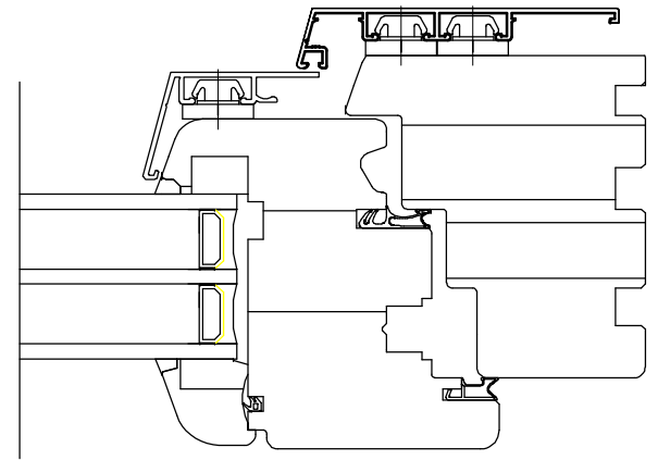
B A-2 Patio Door - Horizontal Section
