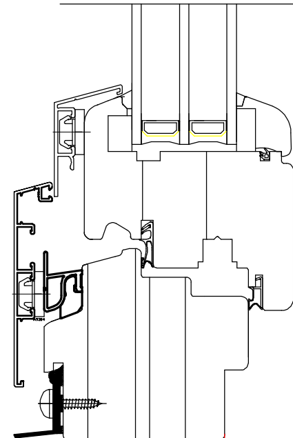
A A-3 Patio Door - Vertical Section
