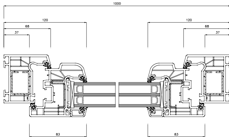
Schnitt S2(5:1)
