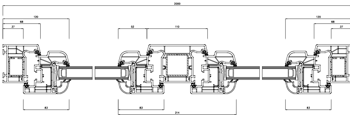
Schnitt S2(5:1)
