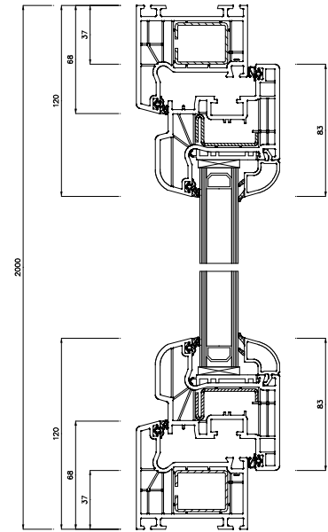
Schnitt S1(5:1)
