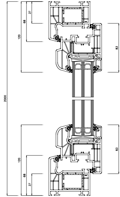
Schnitt S1(5:1)
