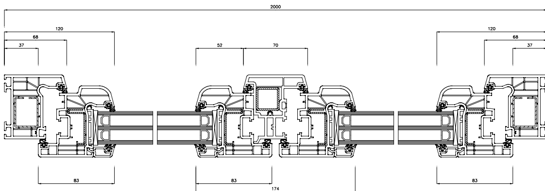
Schnitt S2(5:1)
