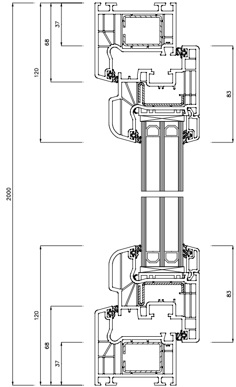
Schnitt S1(5:1)
