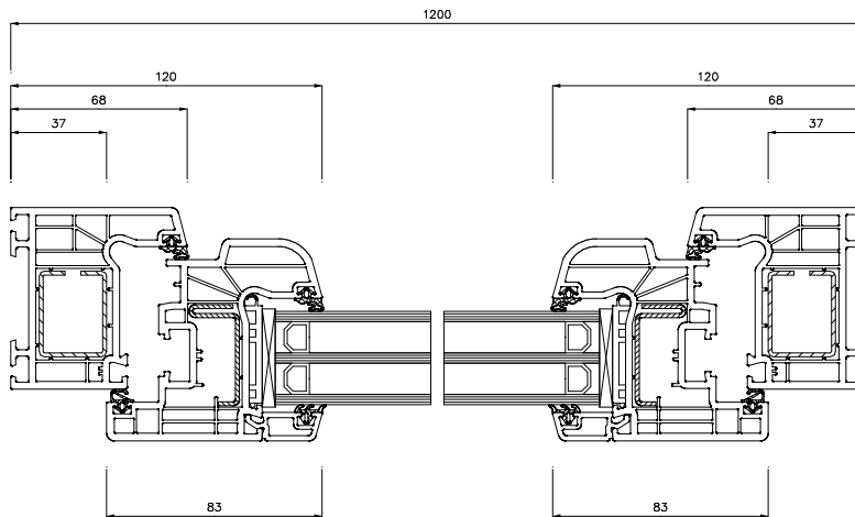
Schnitt S2(5:1)
