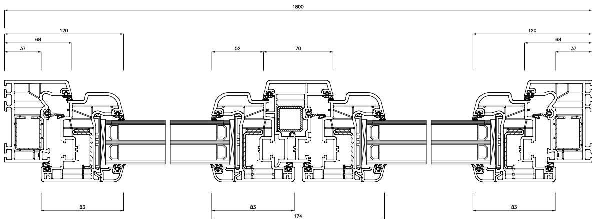
Schnitt S2(5:1)
