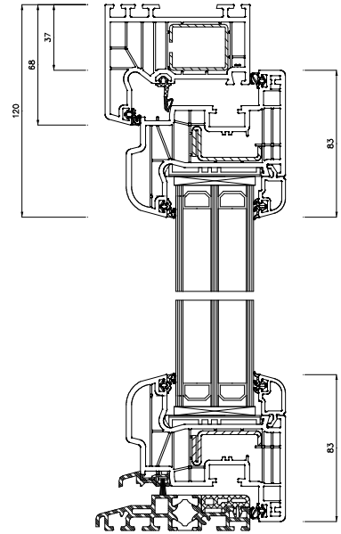
Schnitt S1(5:1)
