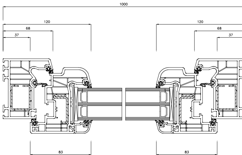
Schnitt S2(5:1)
