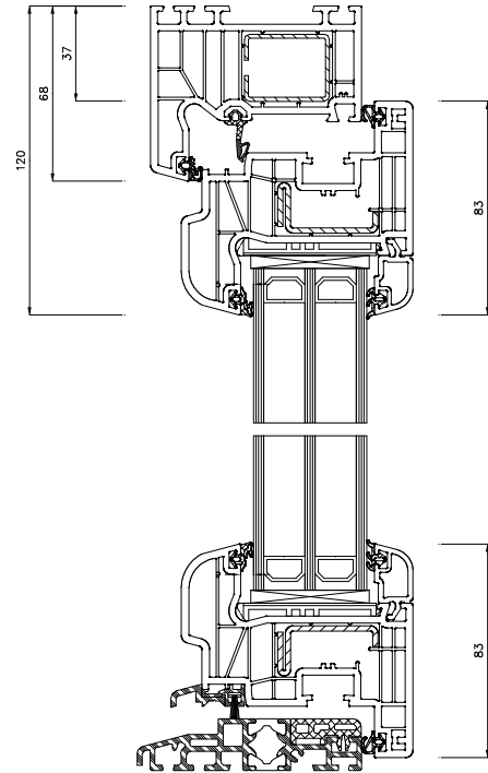
Schnitt S1(5:1)
