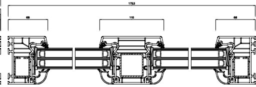
Schnitt S2(5:1)
