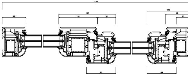
Schnitt S1(5:1)
