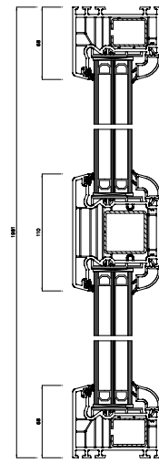
Schnitt S3(5:1)
