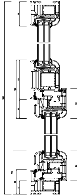
Schnitt S4(5:1)
