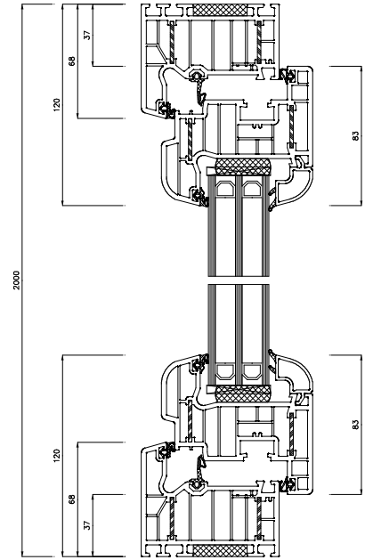
Schnitt S1(5:1)
