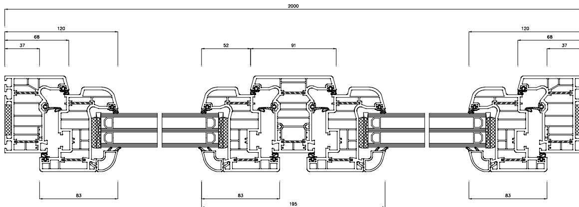
Schnitt S2(5:1)
