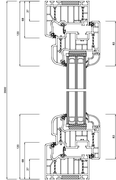
Schnitt S1(5:1)
