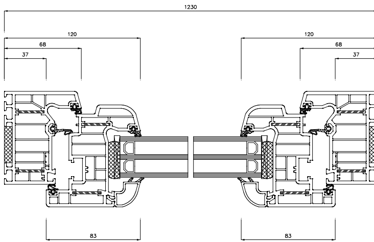
Schnitt S2(5:1)
